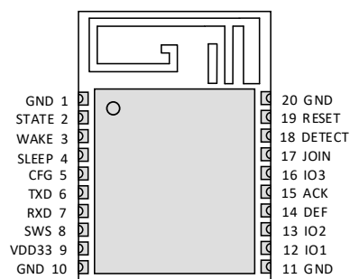
图 3.1 ZM82P0 系列模组引脚定义
