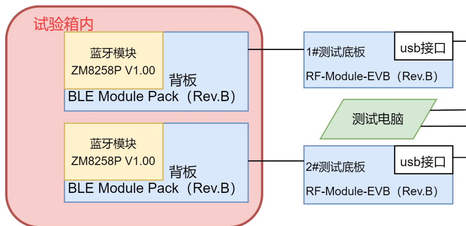
图 2 试验配置框图
