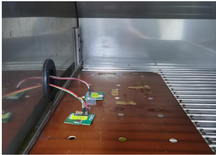
图 3 样机环境试验
