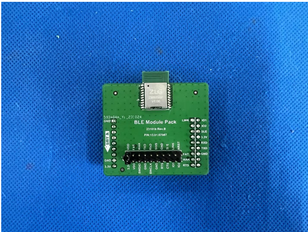
图 7 测试底板图
