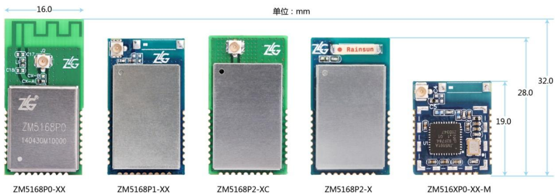
图 1.1 ZM516X 产品外观图
