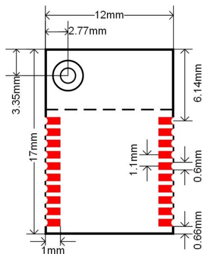
图 5.1 模块尺寸
