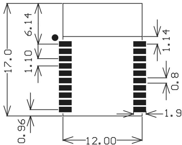
图 5.2 PCB 推荐封装
