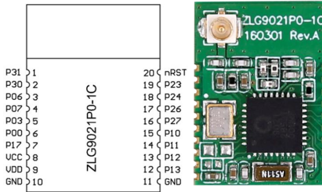
图 2.1 模块引脚图
