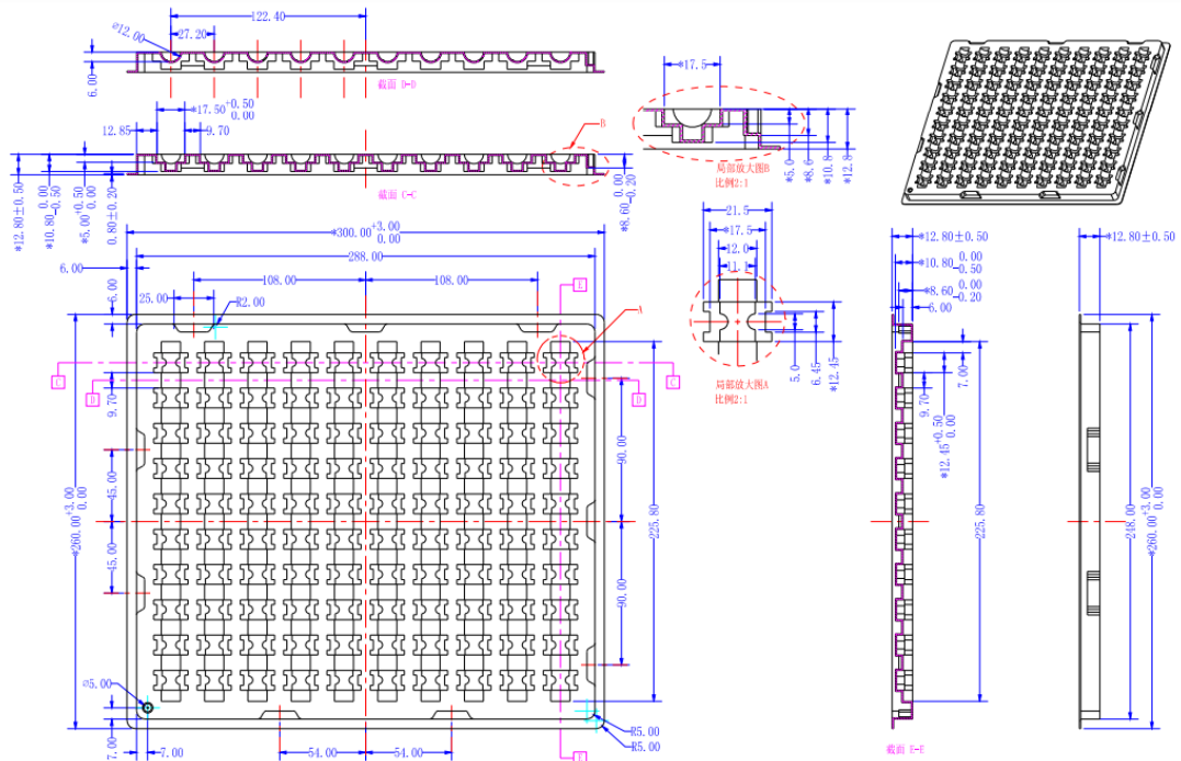
图 6.1 托盘尺寸
