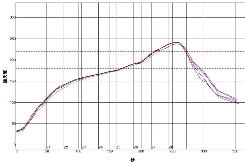
图 7.1 回流焊温度曲线图
