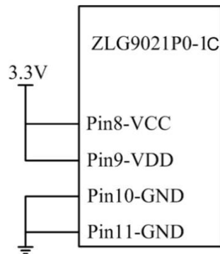
图 4.1 典型应用电路
