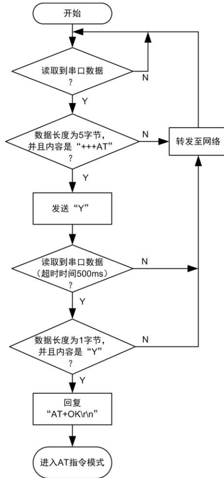
图 8.3 进入 AT 指令模式的处理流程
