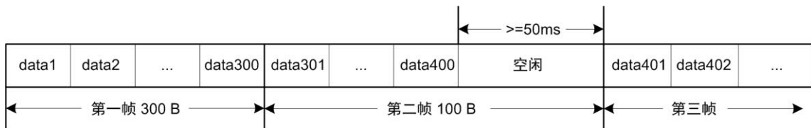
图 4.4.2 串口分帧示意图
