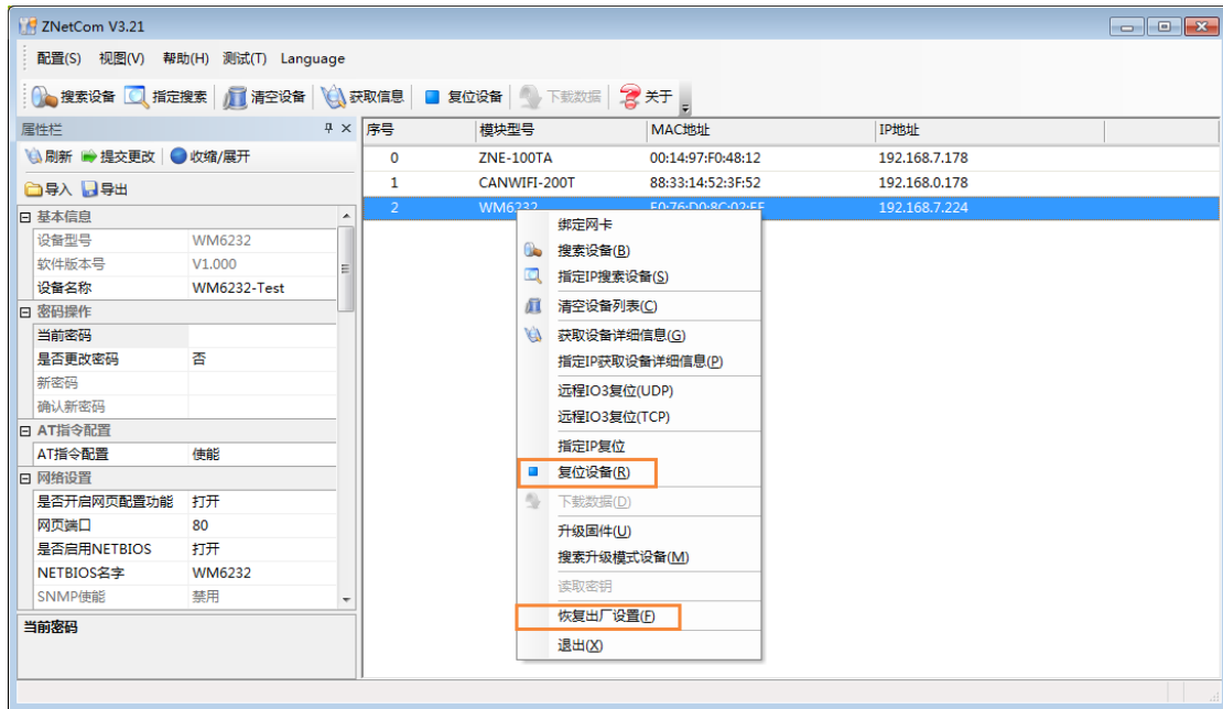
图 7.6 右键菜单
