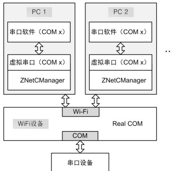
图 4.4.6 虚拟串口通信方式
