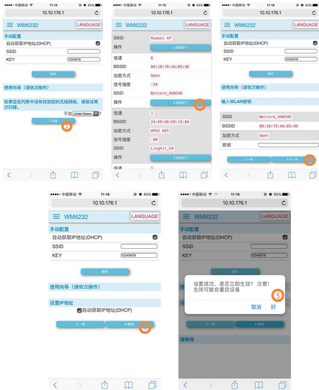
图 5.5 设置向导
