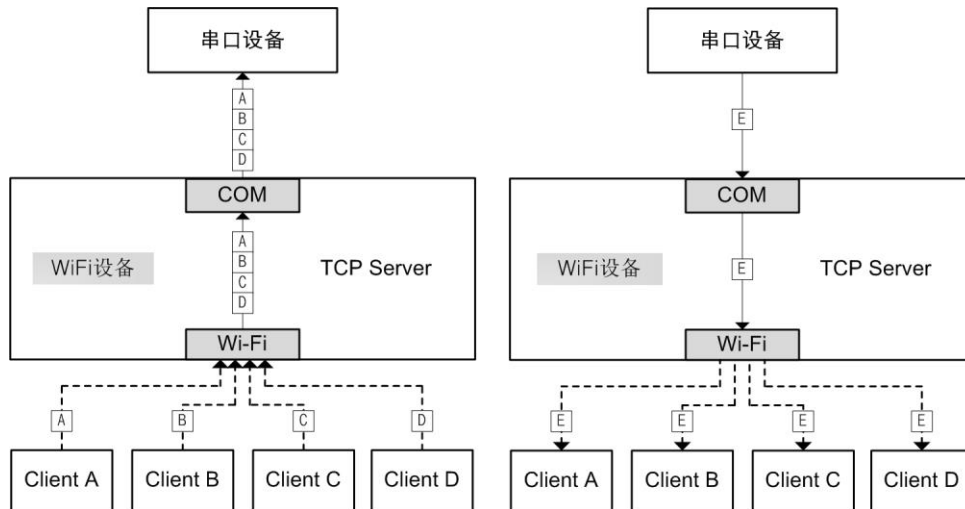
图 4.4.3 TCP Server 模式通信方式
