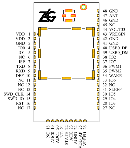
引脚分布图
