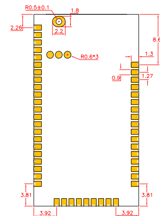
BOTTOM视图
