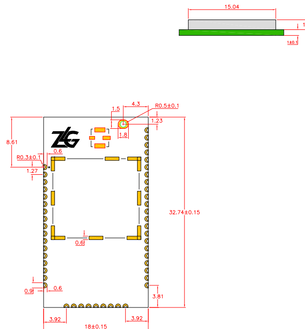
TOP视图
