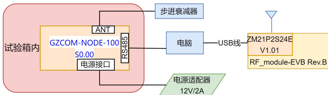
图 2 试验配置框图
