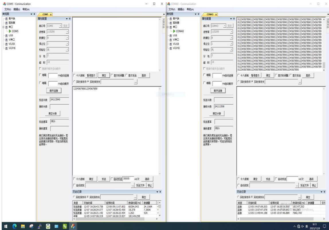
图 13 样机在湿热试验第一次检查功能正常
