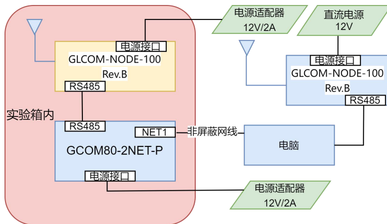
图 2 试验配置框图
