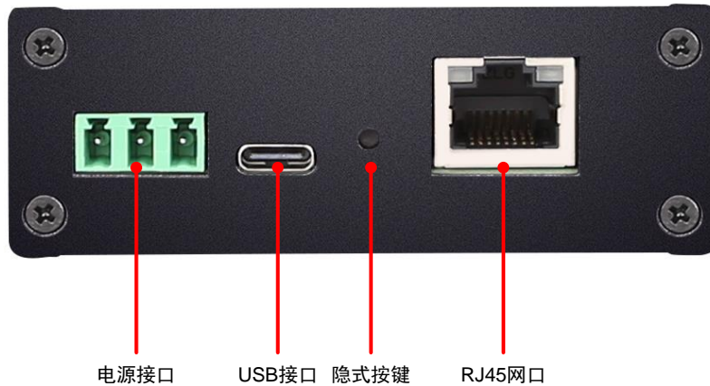
图 2.4 底部接口定义示意图
