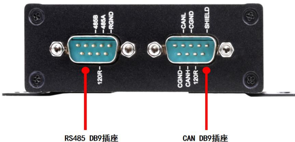
图 2.1 产品顶部图
