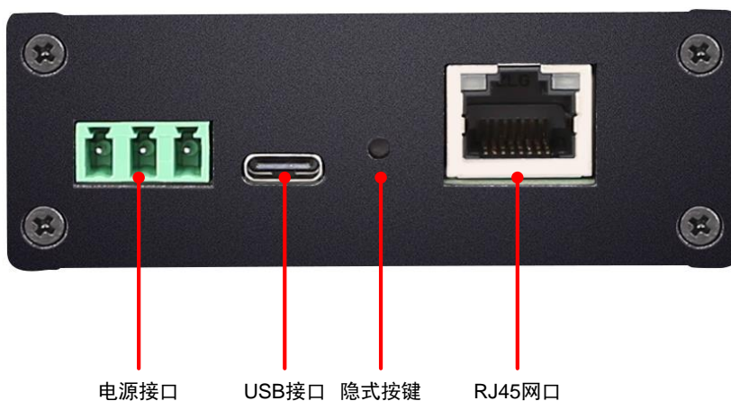
图 2.2 产品底部图
