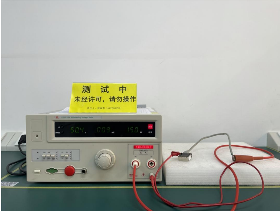
图 7 抗电强度试验
