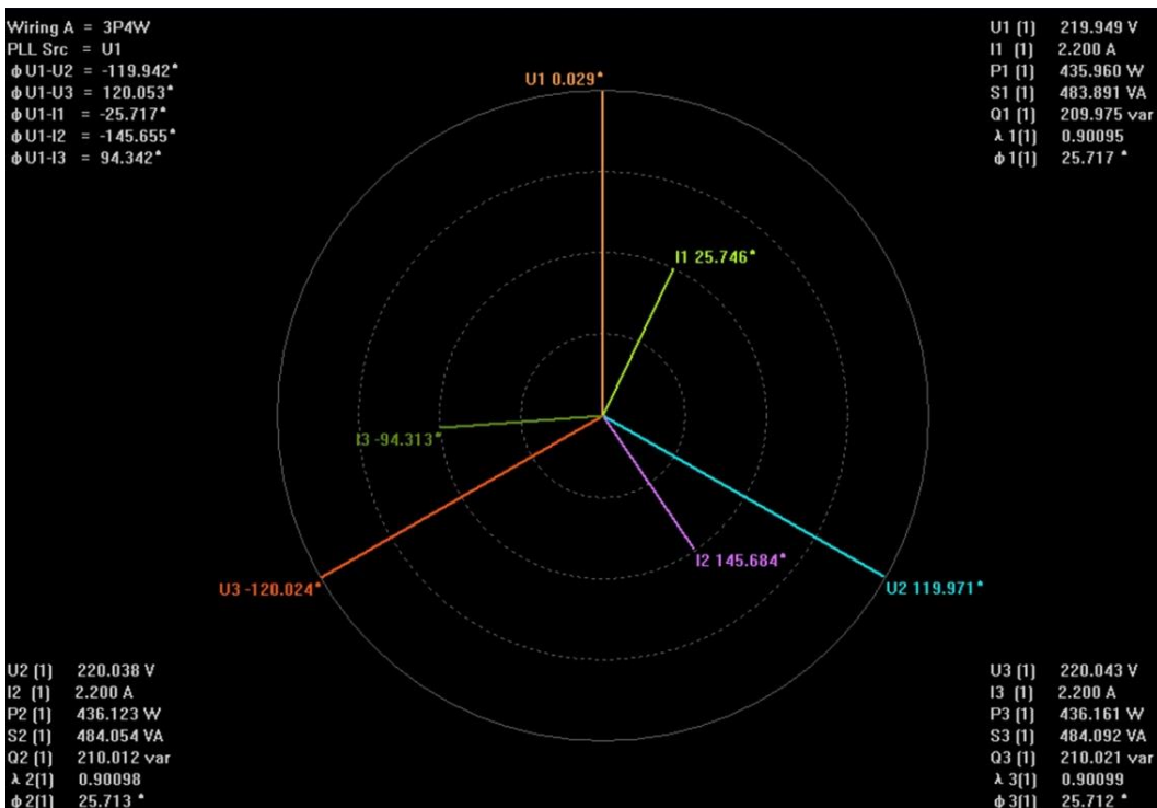
图 2.13 向量显示
