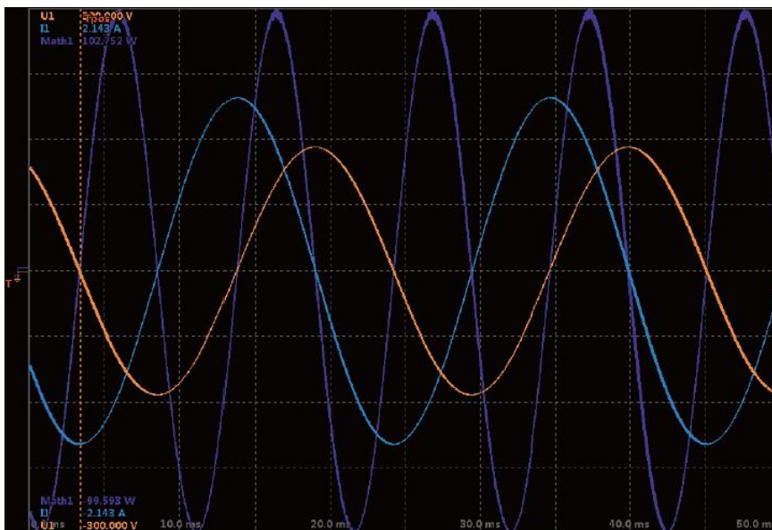
图 2.17 波形运算
