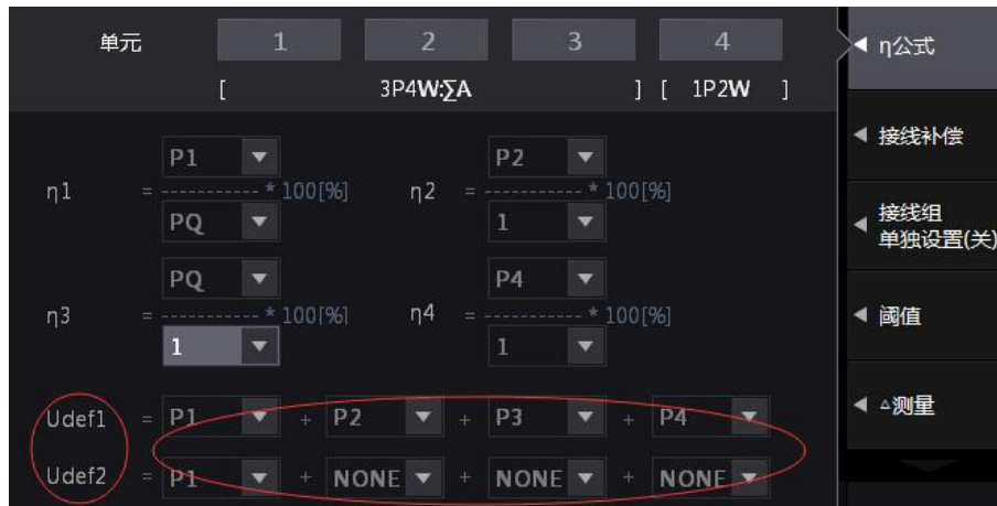
图 4.27 效率运算参数设定
