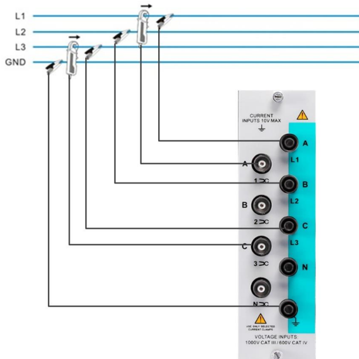
图 4.52 3P3W-2-Element
