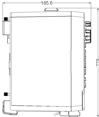
图 7.3 尺寸图 3
