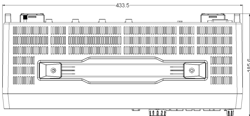
图 7.1 尺寸图 1
