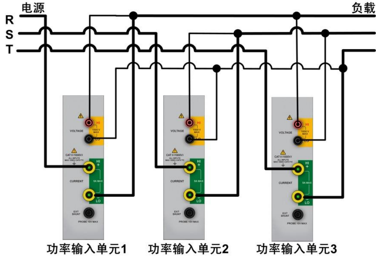
图 4.46 3P3W (3 电压 3 电流表法) 下光伏逆变器综合测试仪接线示例
