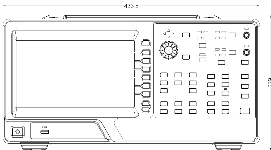
图 7.2 尺寸图 2
