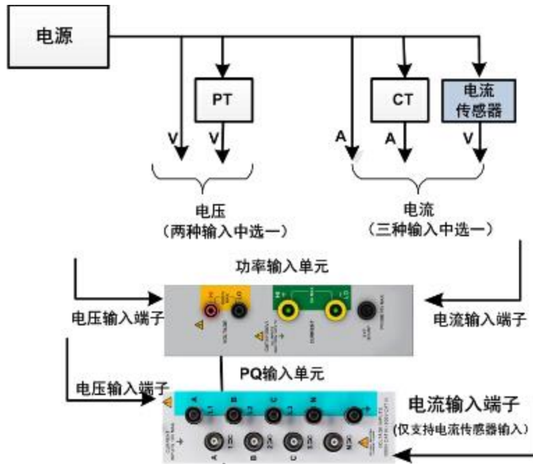
图 2.20 输入信号到输入单元
