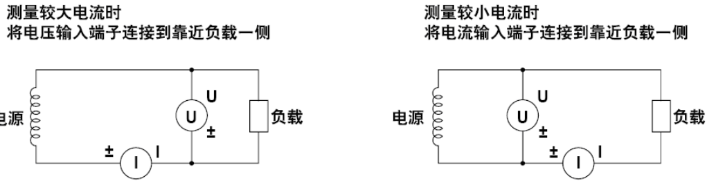
图 4.34 测量电压和电流的大小对测量的影响
