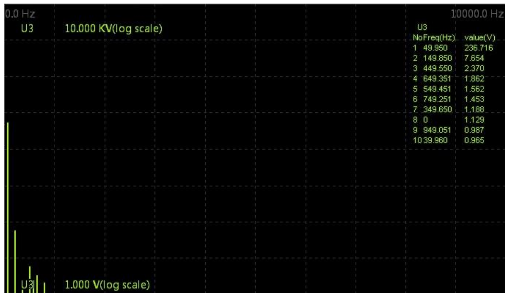
图 2.10 FFT 波形显示
