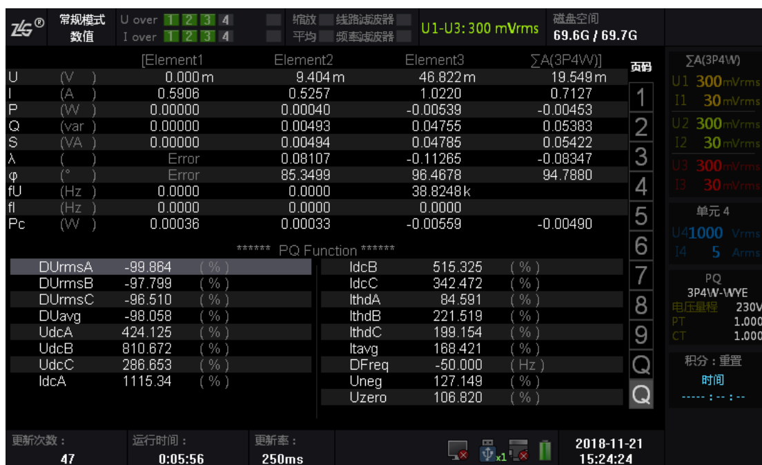
图 2.3 PQ 数值显示界面-2
