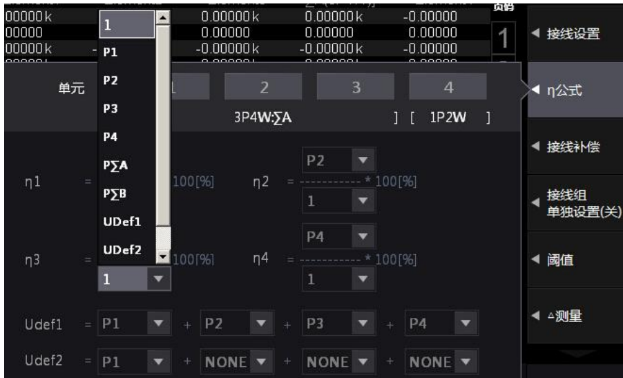
图 4.26 效率公式分子/分母配置
