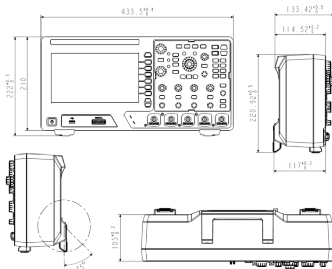
图 3.1 ZDS2000B 示波器尺寸图
