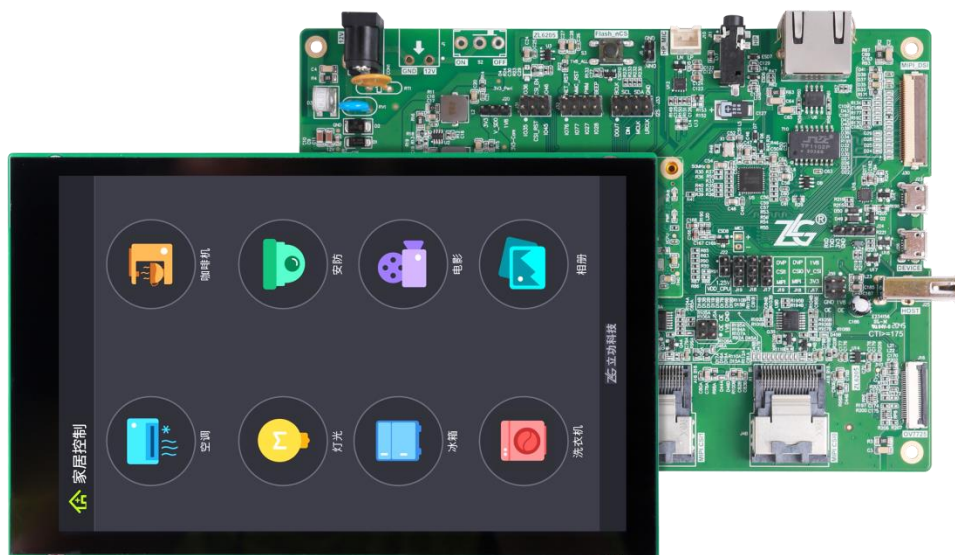
图 1 ZMP1107_EVB 评估套件示意图
