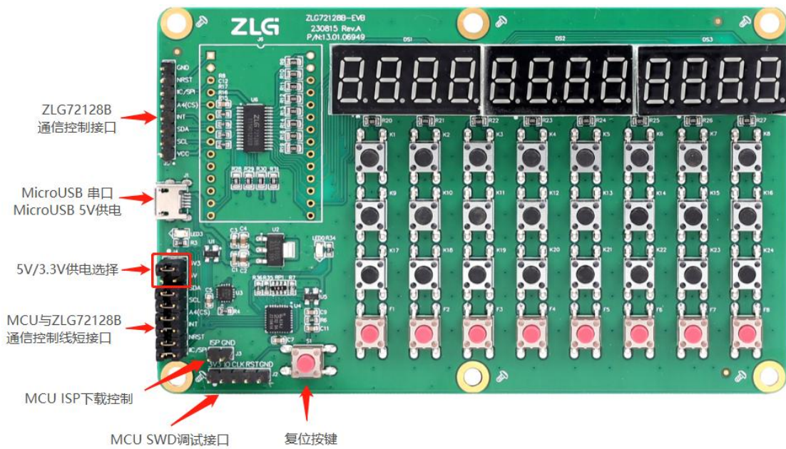
图 1.2 接口说明
