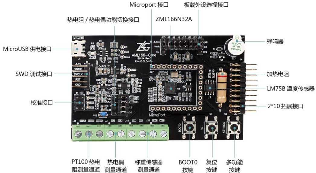
图 1.1 AML166-Core 开发平台
