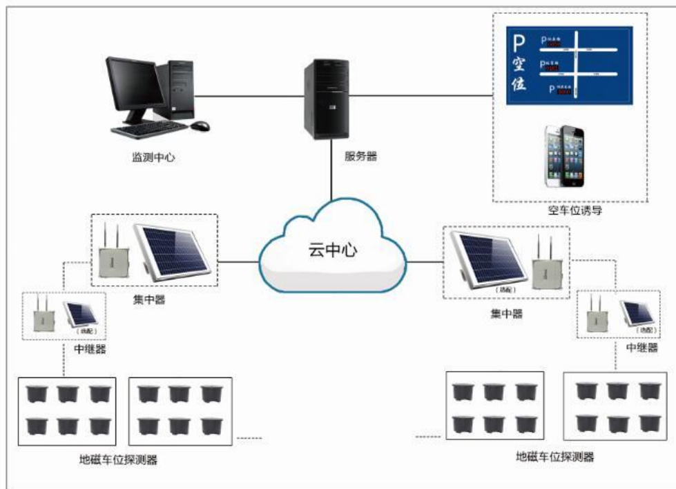
图 1.1 系统架构图
