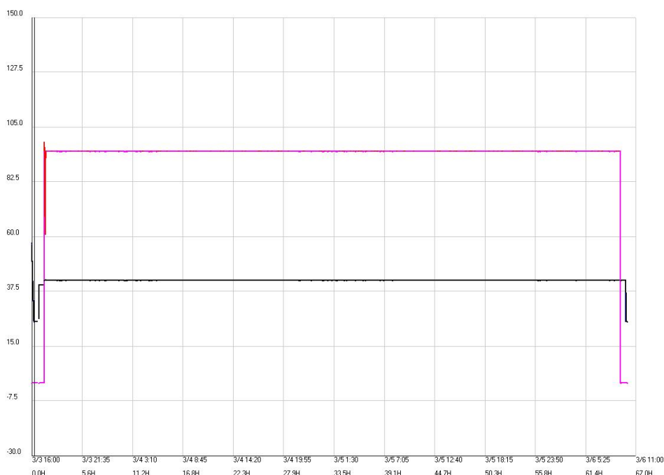
备注: THMP_PV: 实际温度, THMP_SP: 温度设定值; HUMI_PV: 实际湿度, HUMI_SP: 湿度设定值
