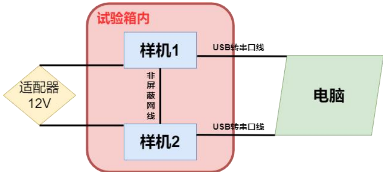
图 2 试验配置框图
