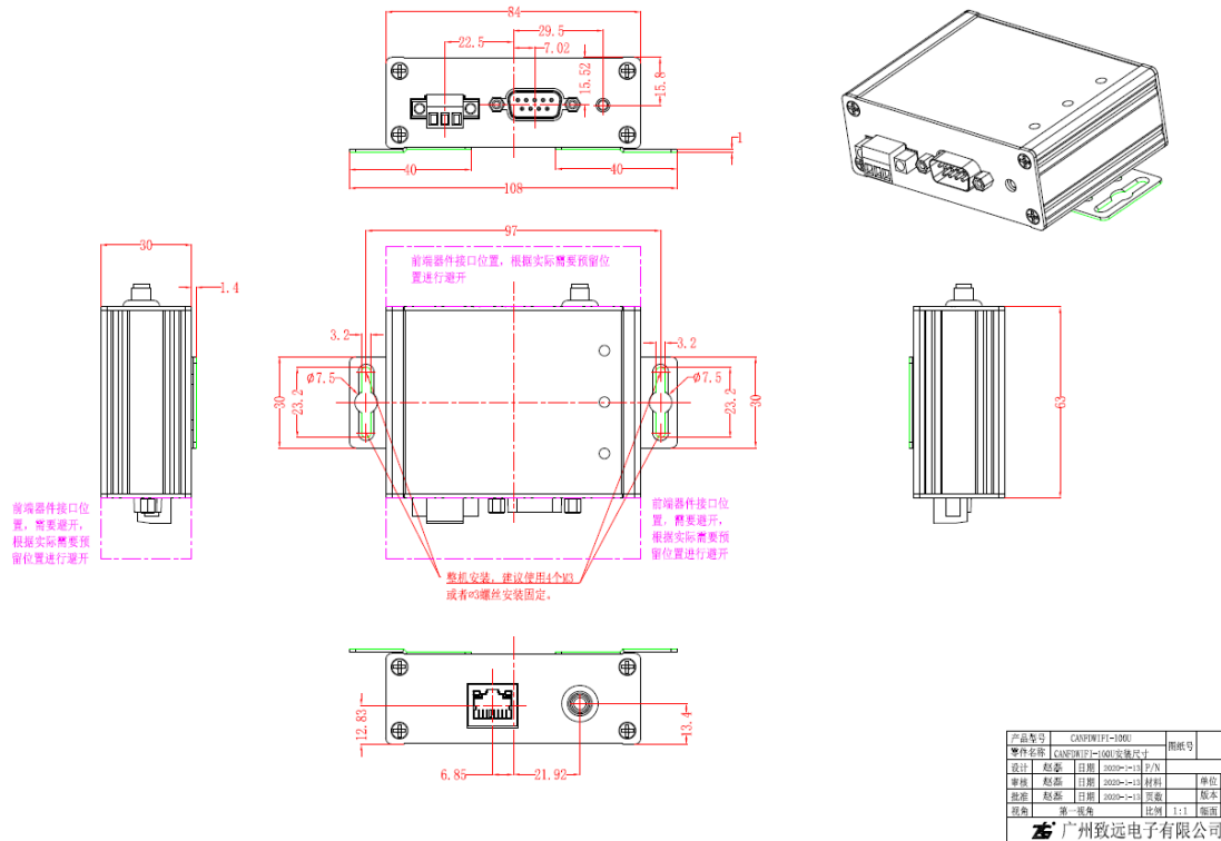
图 3.1 主机尺寸图
