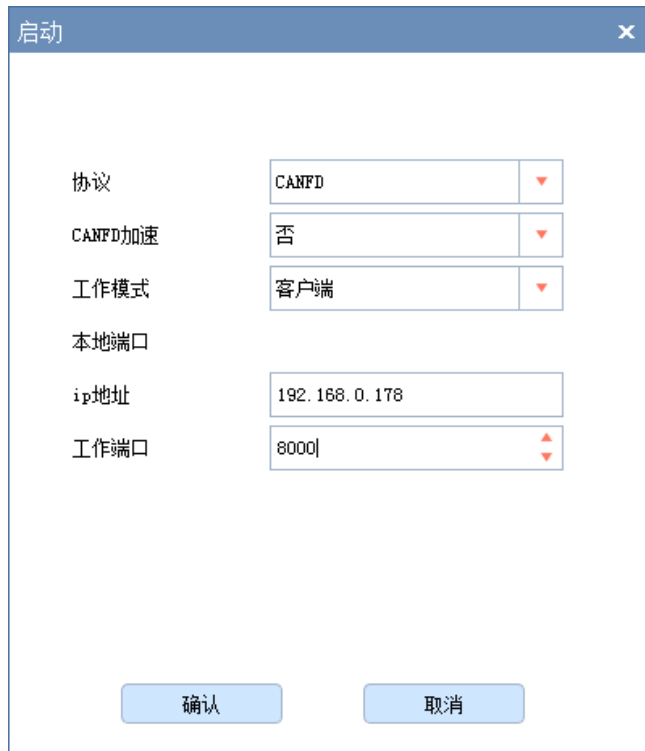
图 5.8 启动 CANFDNET-TCP 客户端界面
