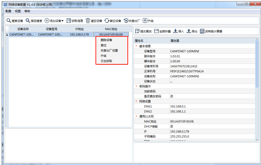
图 6.1 网络配置工具设备功能显示
