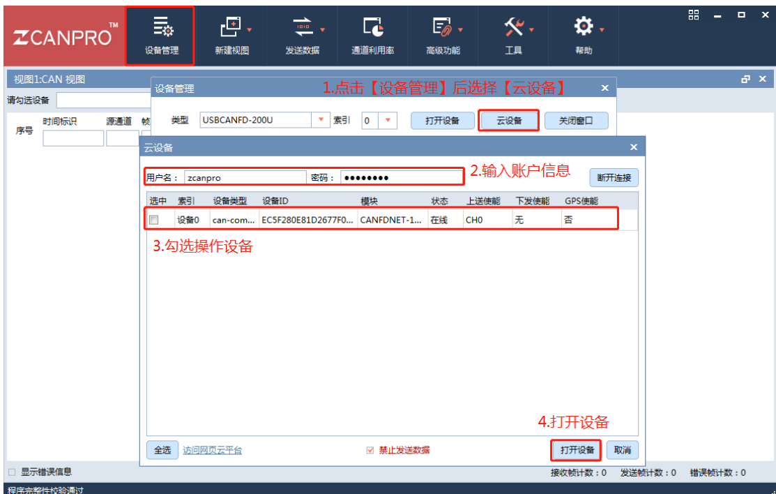
图 6.11 ZCANPRO 打开云设备
