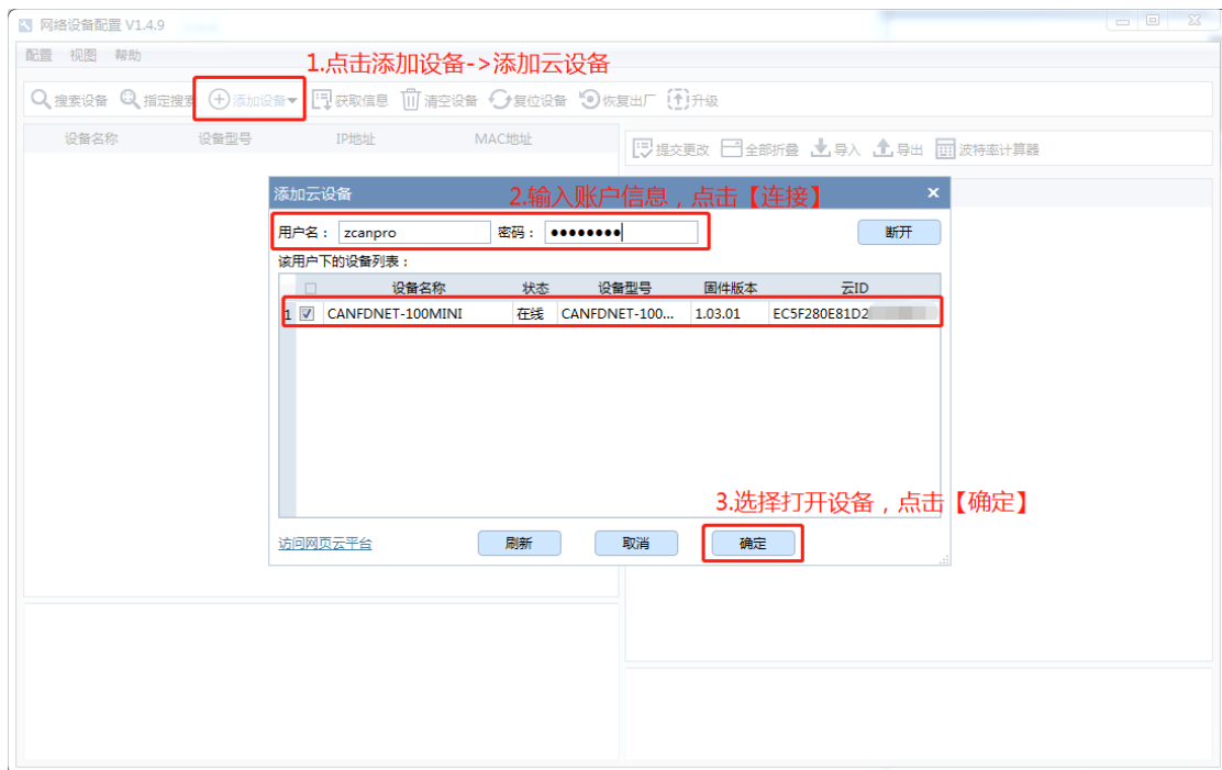
图 6.9 打开云设备操作示意图
