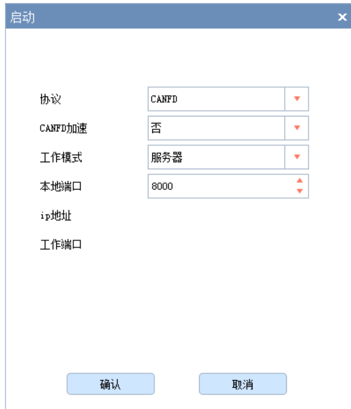
图 5.10 启动 CANFDNET-TCP 服务器界面
