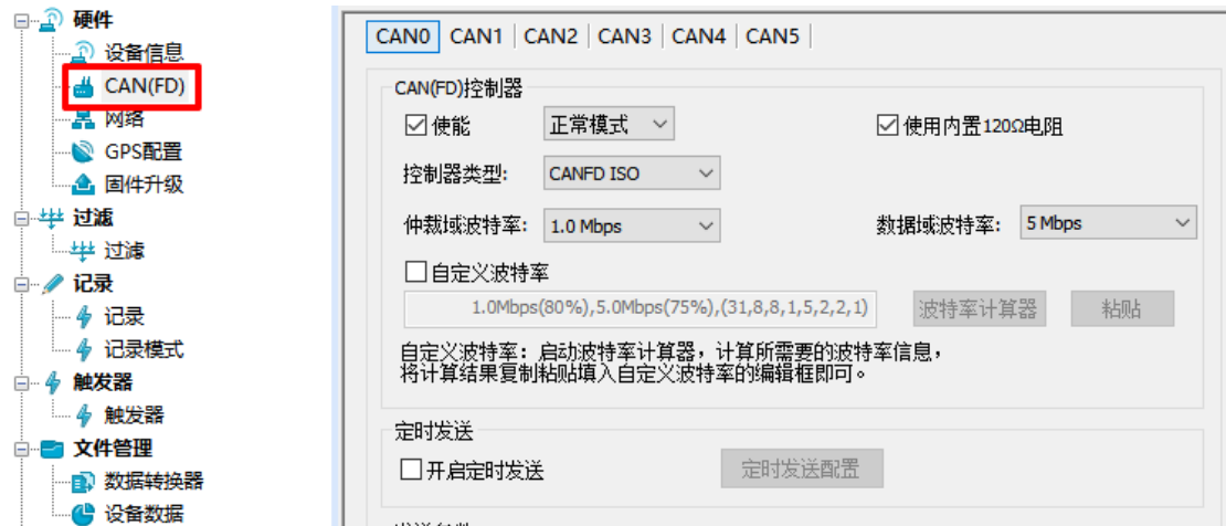
图 5.3 CAN (FD) 通道配置界面
