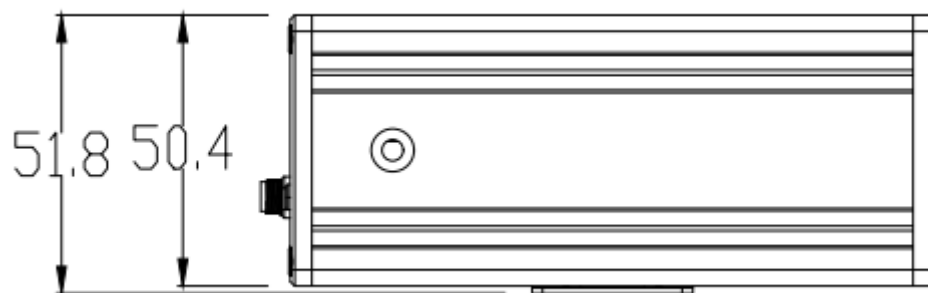
图 3.2 主机尺寸图二
