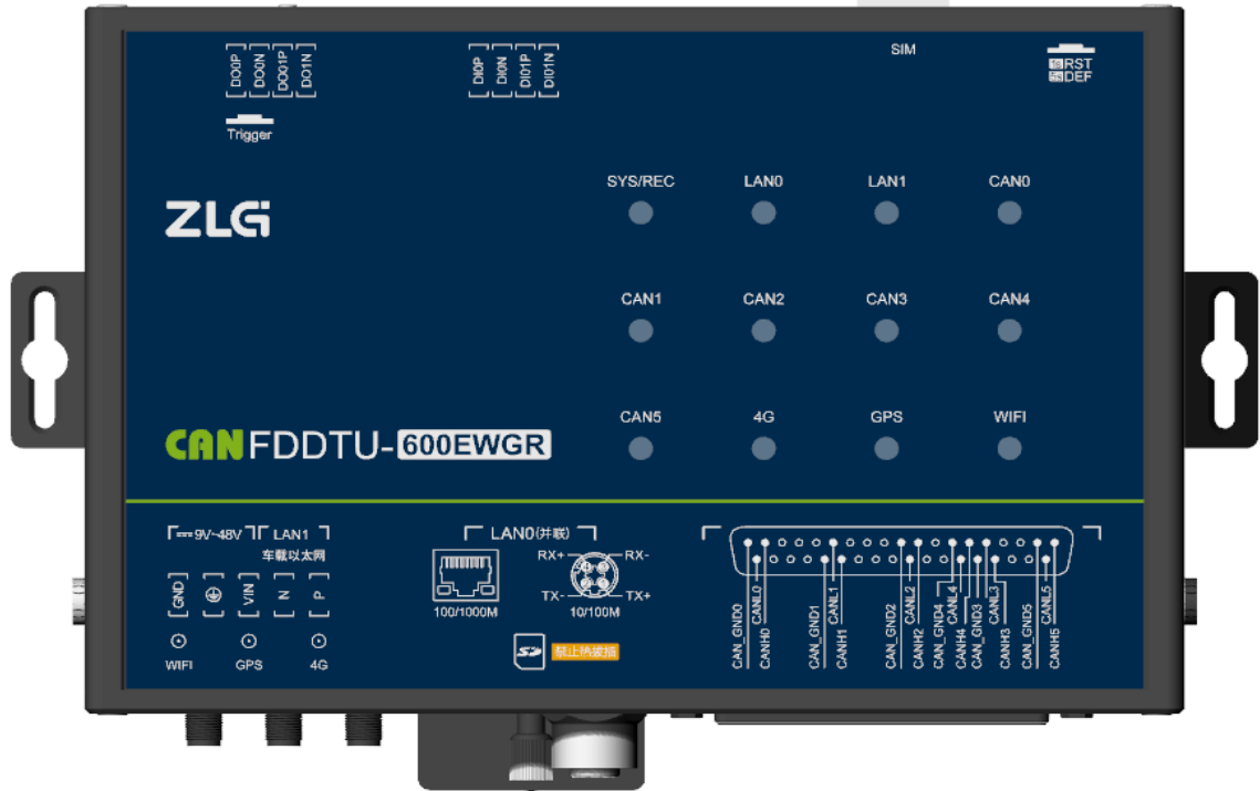
图 4.1 面板布局
