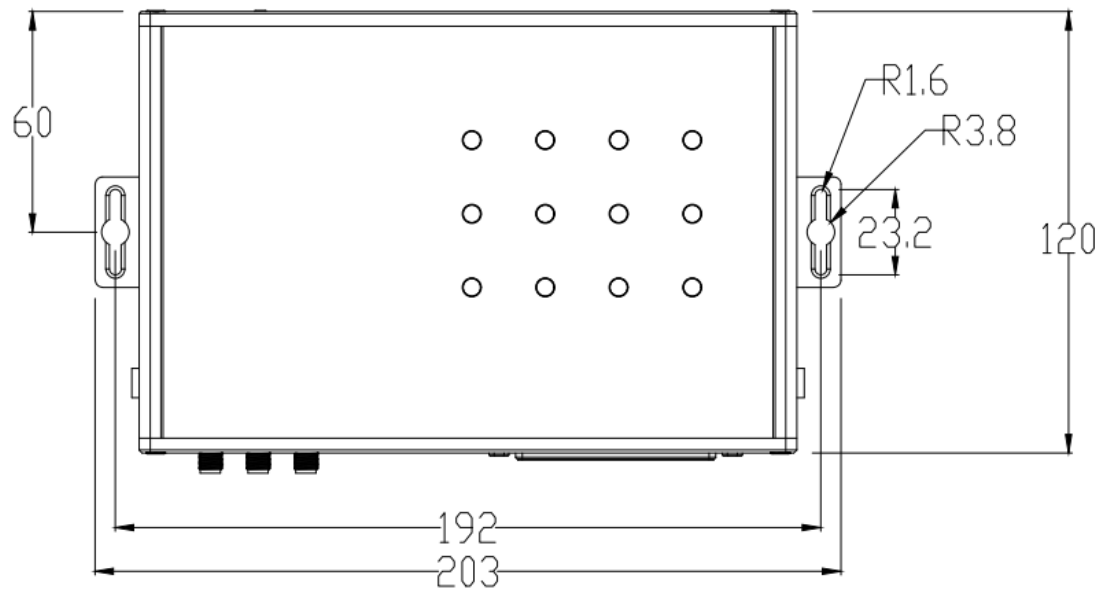
图 3.3 安装方式
