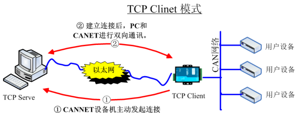
图 5.2 TCP Client 模式通讯示意图
