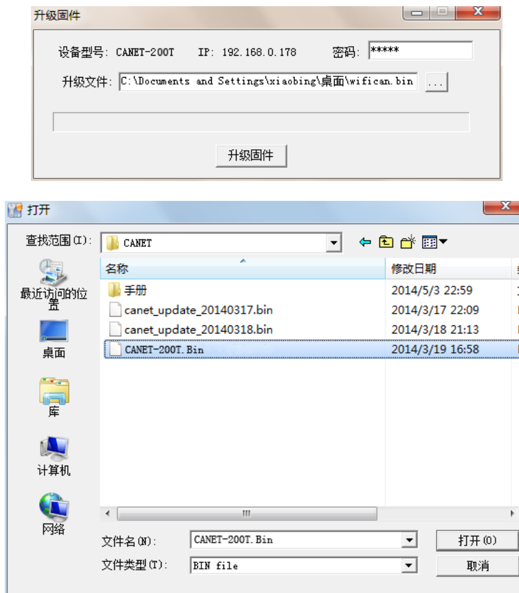
图 6.15 固件升级界面
