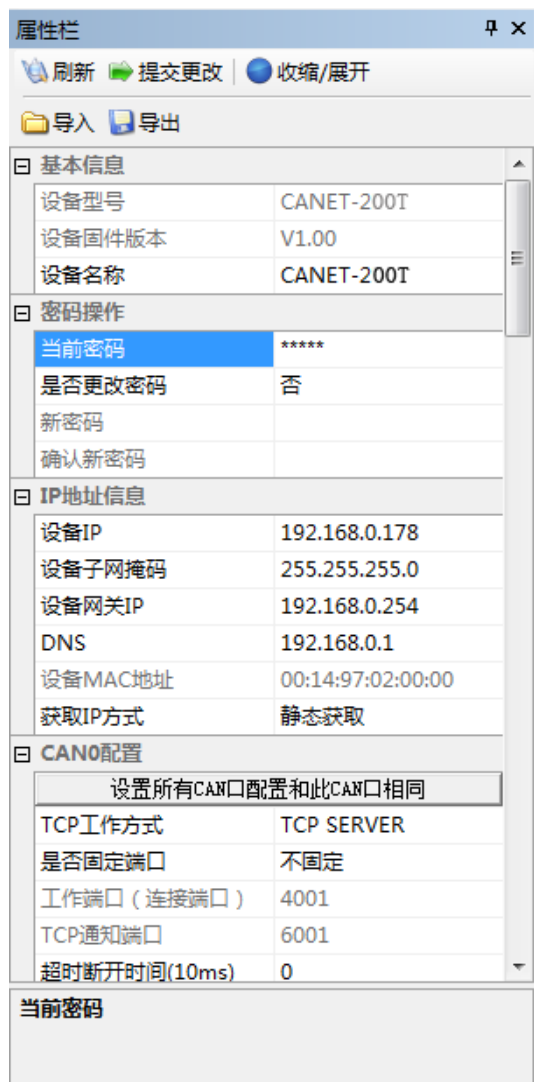
图 6.10 修改 CANET 设备配置
