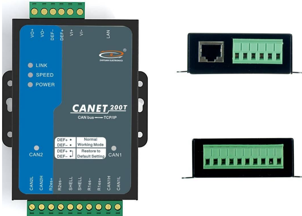
图 2.1 CANET-200T 外观图
