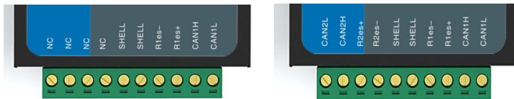
图 2.5 CANET-100T(左)和 CANET-200T(右)的 CAN 口外观图
