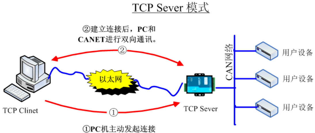
图 5.1 TCP Server 模式通讯示意图
