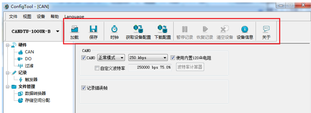
图 4.8 设备有效
