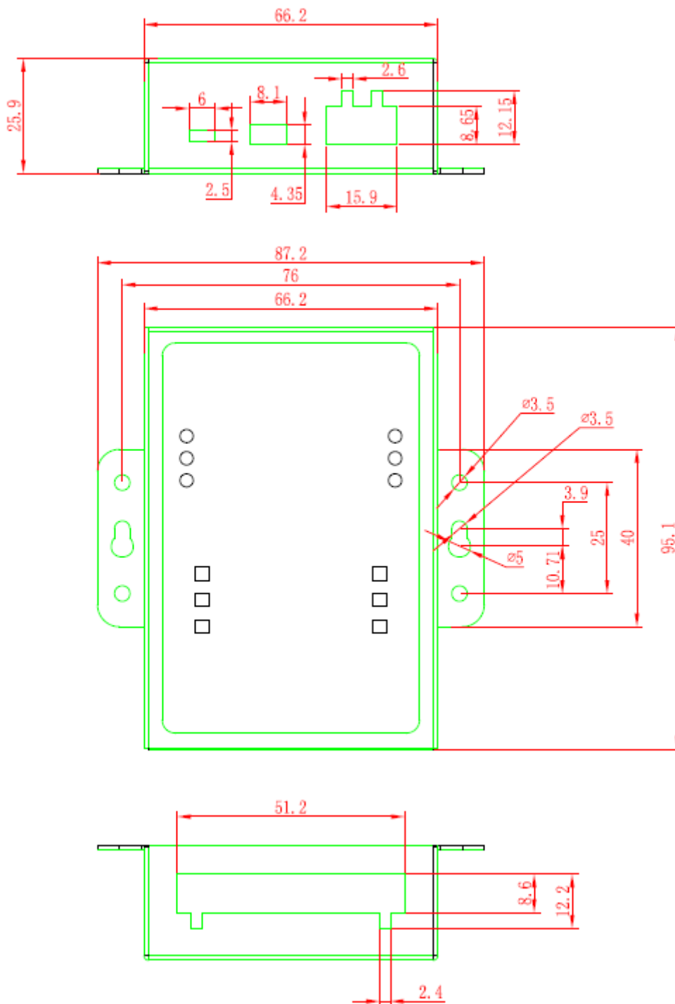
图 7.1 产品尺寸图
