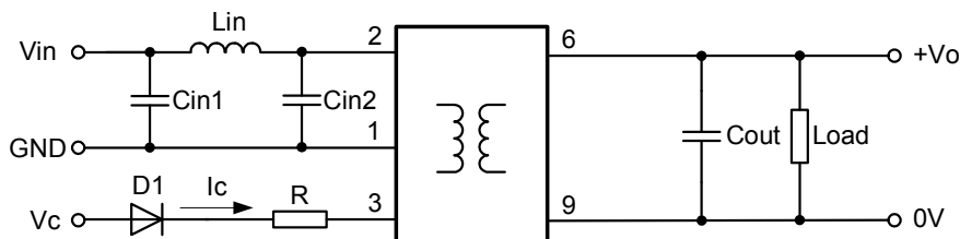
图 1 应用电路图
