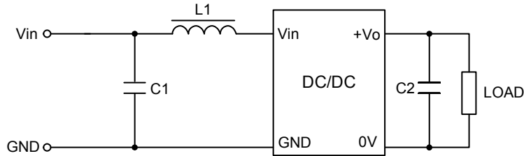
图 2 EMC 推荐应用电路
