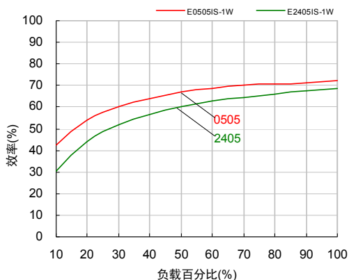
效率与负载关系曲线图(输入标称电压)
