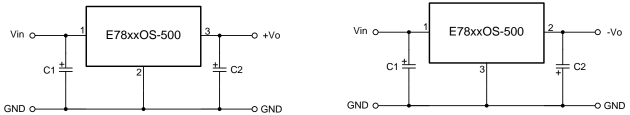
图 1 正输出（左）和负输出（右）应用电路图
